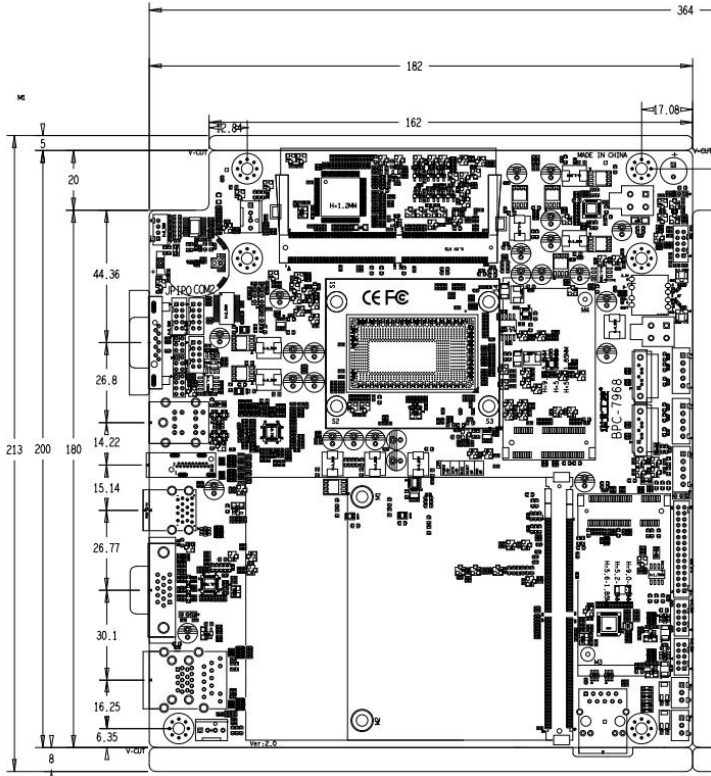
BPC-7968 接口位置和尺寸图
