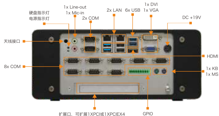
BIS-6910E接口
